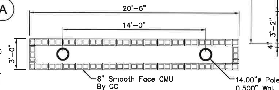
SECTION B SCALE: \frac{3}{8} " = 1'-0"
