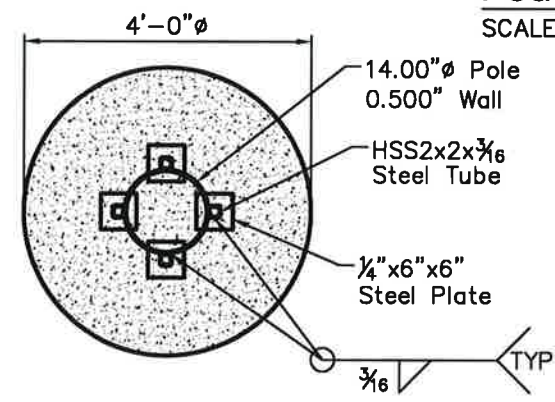
SECTION A SCALE: \frac{3}{8} " = 1'-0"
